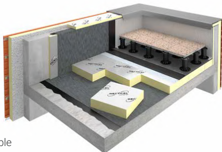
Protection lourde terrace inaccessible
